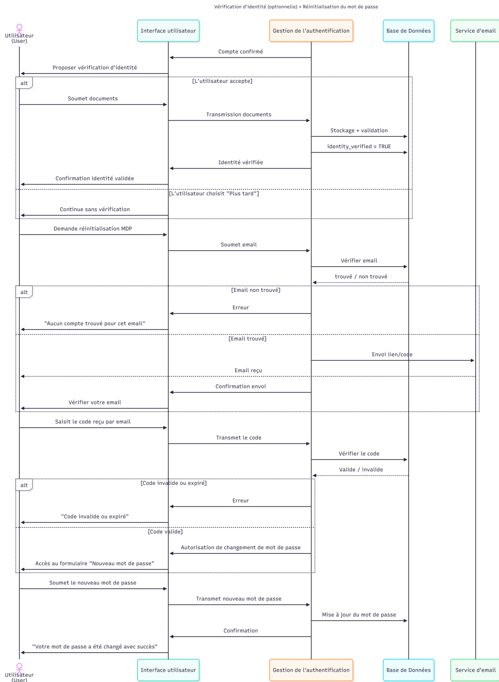
Diagramme de séquence qui décrit le processus de vérification des informations d'un utilisateur
